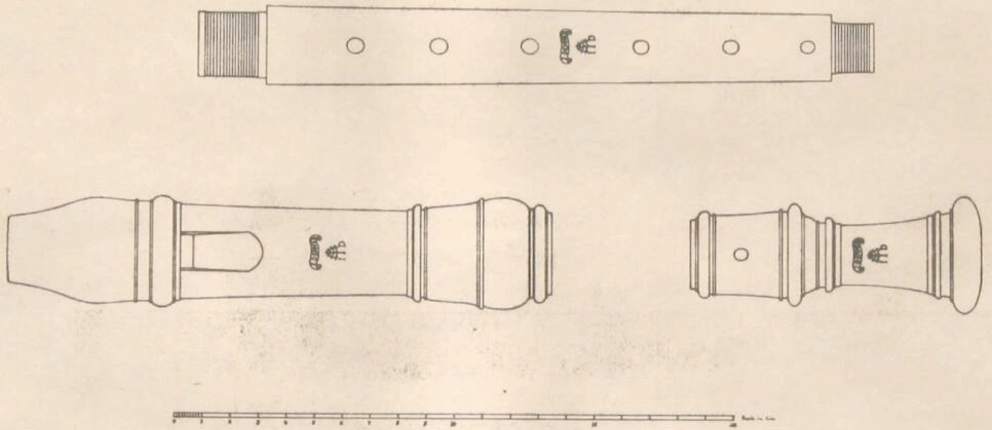
FIG. 2 Jacob Denner Treble Recorder, Musikhistorisk Museum, Copenhagen. (F. von Huene, del.)
